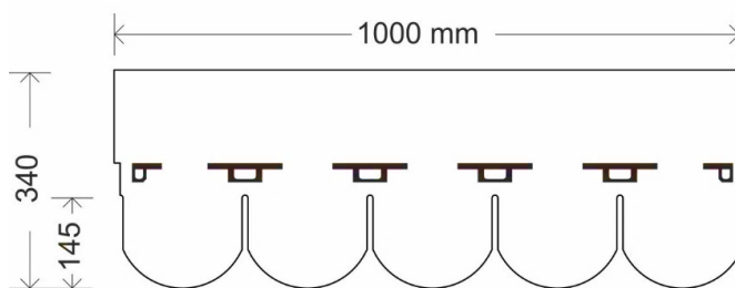
Fig. 1 - Dimensioni tegola Traditional
