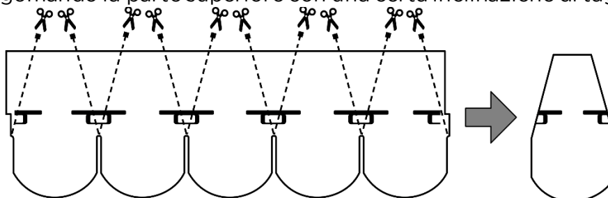
Fig. 10 - Preparazione elementi colmo
