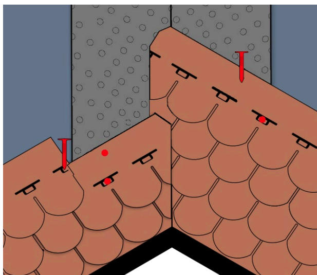
Fig. 13 - Posa tegole sul compluvio
