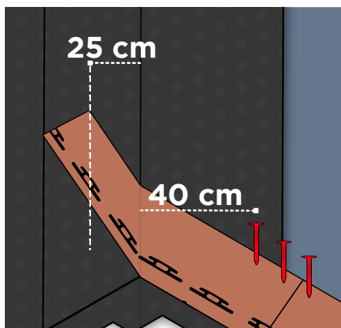
Fig. 12 - Posa tegole sul compluvio
