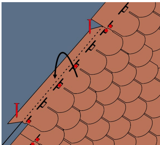
Fig. 9 - Posa delle tegole al colmo
