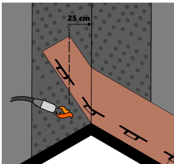
Fig. 20 - Installazione a fiamma delle tegole sul compluvio
