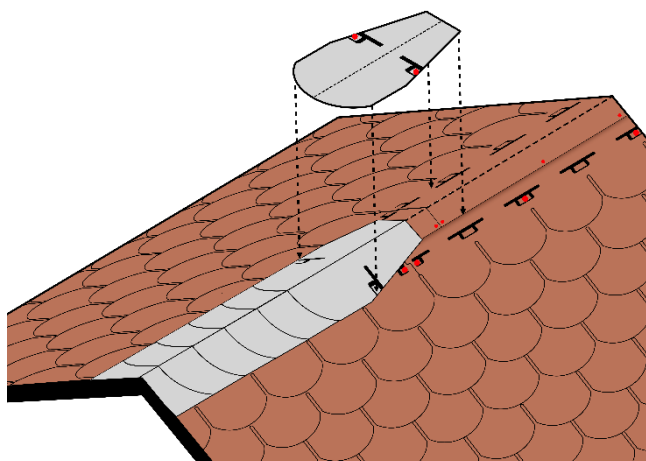
Fig. 11 - Posa elementi colmo
