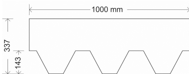
Fig. 1 - Dimensioni tegola Mosaik
