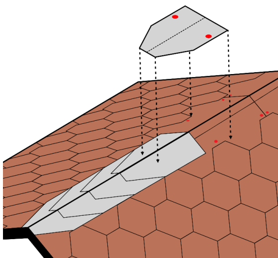
Fig. 11 - Posa elementi colmo
