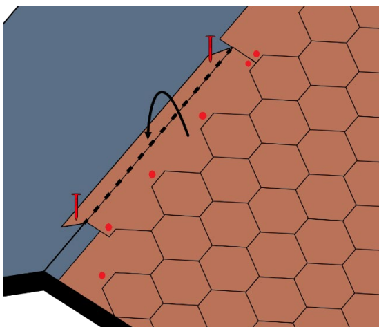
Fig. 9 - Posa delle tegole al colmo
