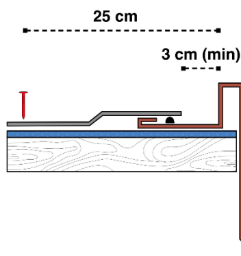
Fig. 4 - Dettaglio lamiera laterale
