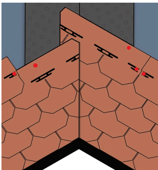
Fig. 13 - Posa tegole sul compluvio
