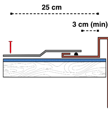
Fig. 4 - Dettaglio lamiera laterale
