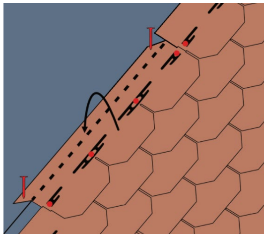
Fig. 9 - Posa delle tegole al colmo
