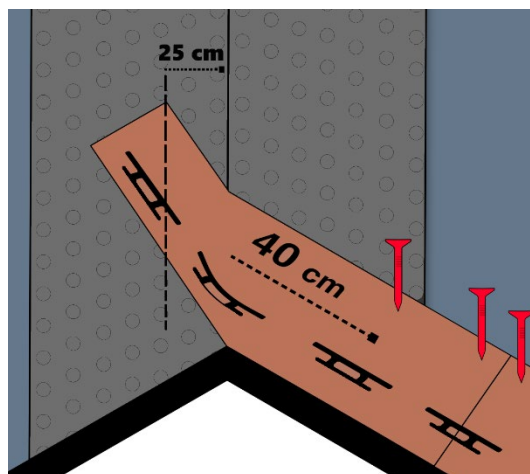
Fig. 12 - Posa tegole sul compluvio
